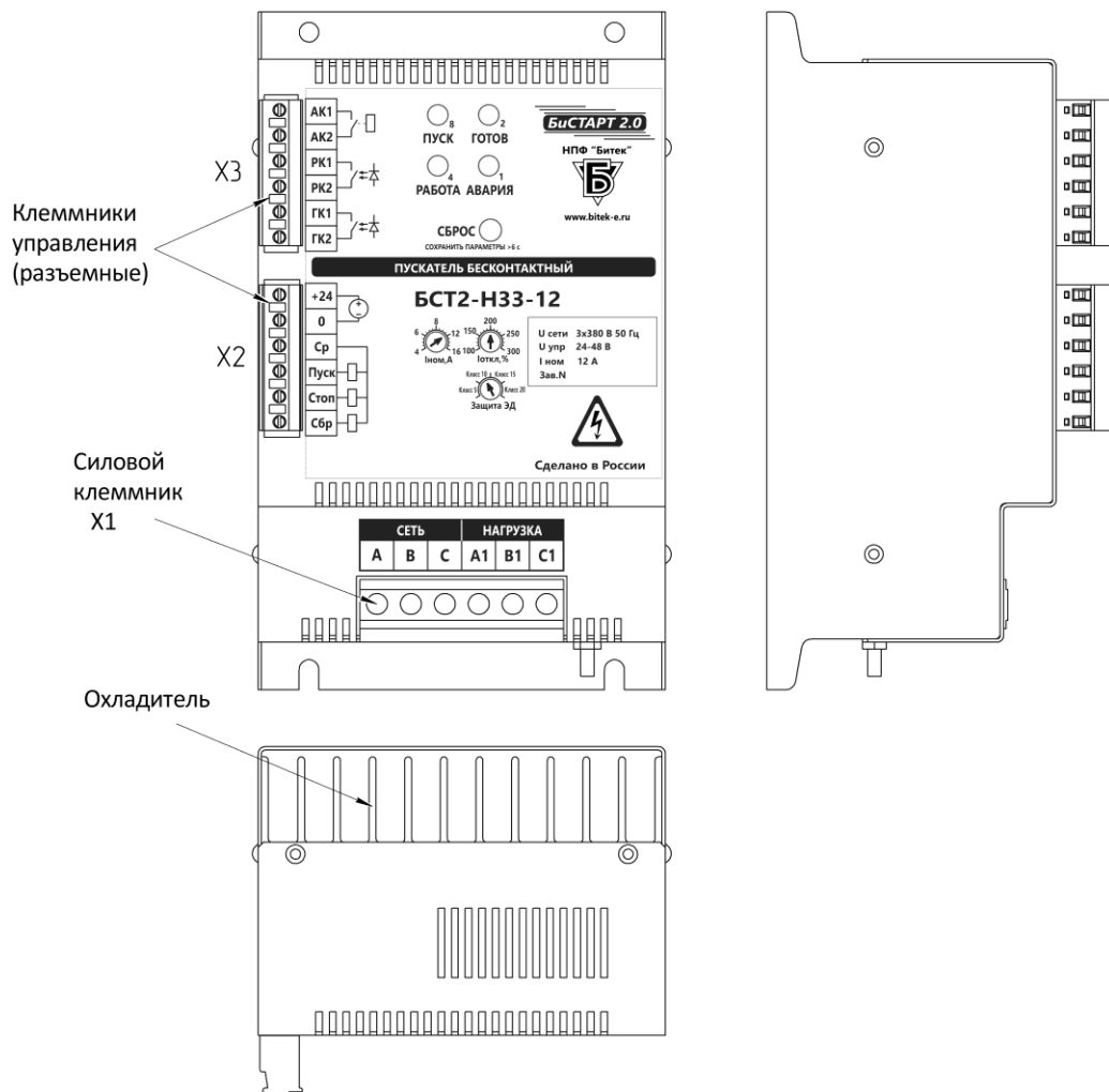
Рисунок 1 - Внешний вид пускателя БСТ2-Н33-12 (см. также Приложение А)
