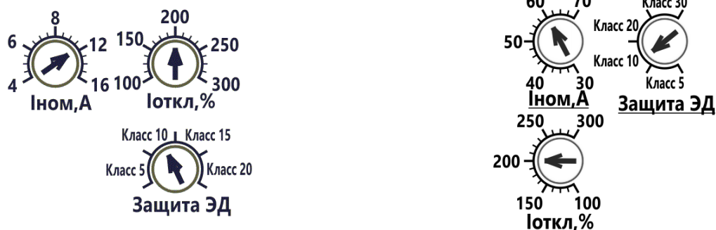
Рисунок 5 Органы настройки БСТ2-НЗ
