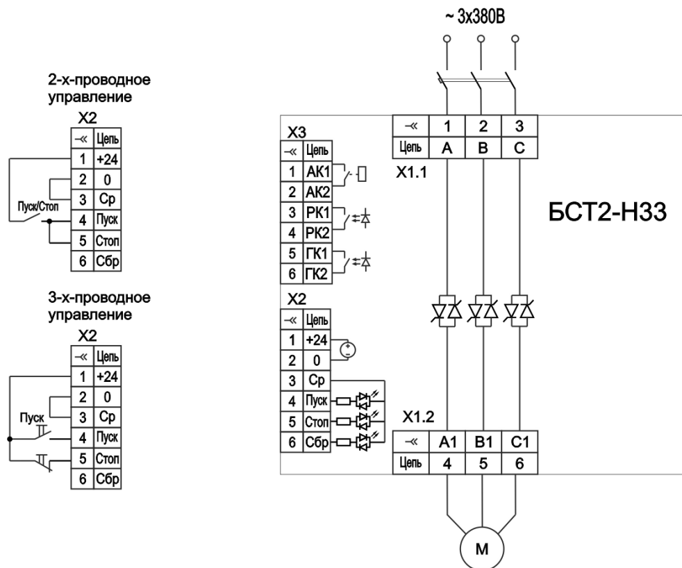
Рисунок 4 – Пример схемы подключения БСТ2-Н33
