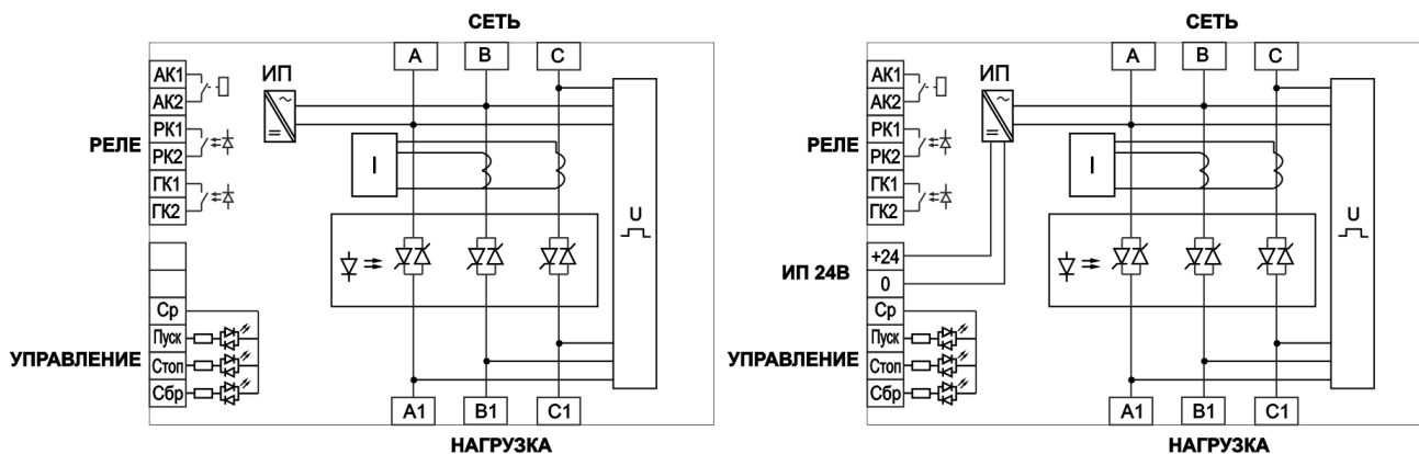
а) БСТ2-Н30, БСТ2-Н31, БСТ2-Н32
